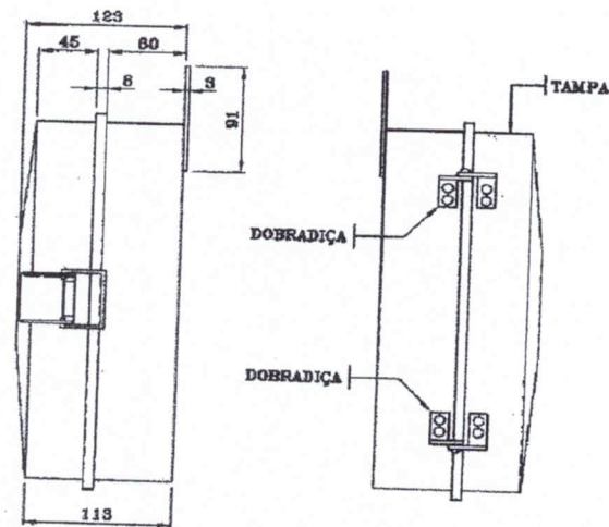
VISTA LATERAL ESQUERDA SEM RELE FOTOELÉTRICO E SEM A BASE DO RELE
