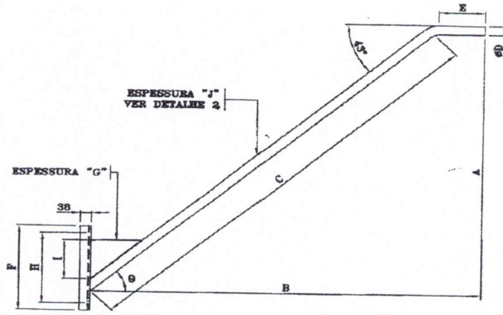
VISTA LATERAL
