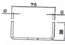
BASE DO BRAÇO CORTE A-A'
