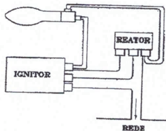
DETALHE 1
