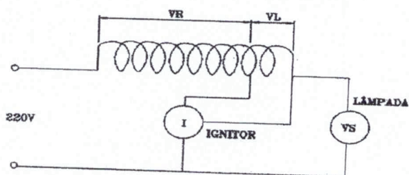
DETALHE 2
